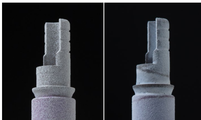
Слева: равномерное нанесение с помощью Renfert-Scanspray extra fine / Справа: неравномерный слой при использовании продуктов конкурентов
